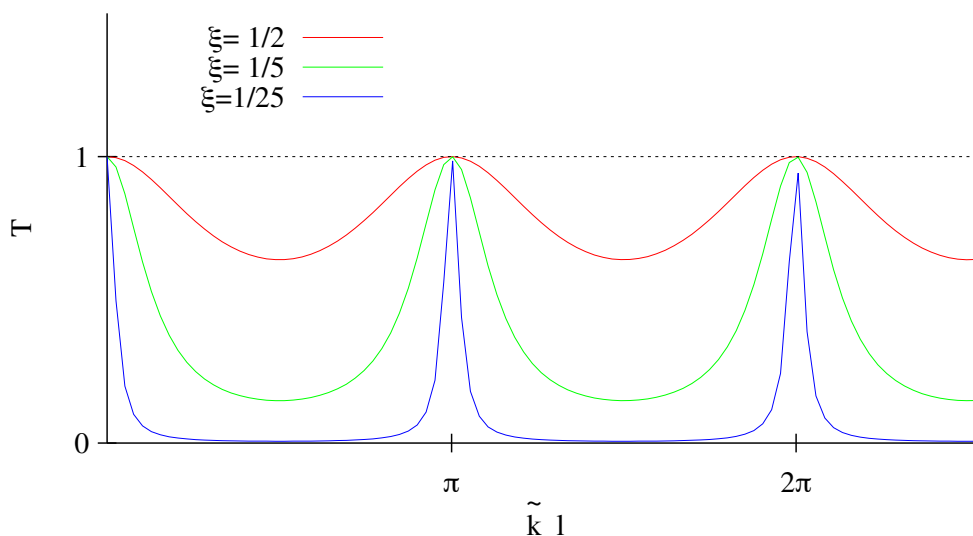
ABBILDUNG 1.12: Transmissionsamplitude T_k für verschiedene Werte von \xi
