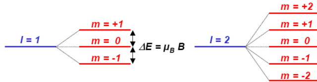
ABBILDUNG 3.3: Darstellung der Niveaufaltung für die Fälle l = 1 und l = 2
