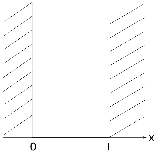
ABBILDUNG 1.7: Unendlich tiefer Potentialtopf
