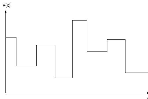
ABBILDUNG 1.6: Stückweise konstantes Potential in einer Raumdimension
