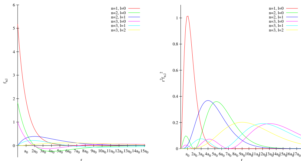
ABBILDUNG 3.2: links: Radialwellenfunktionen bis n = 3 , rechts: zugehörige Wahrscheinlichkeitsdichte. Der Faktor r^2 stammt dabei von der Funktionaldeterminante des Basiswechsels in Kugelkoordinaten.
