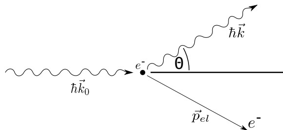
ABBILDUNG 1.2: Compton-Effekt
