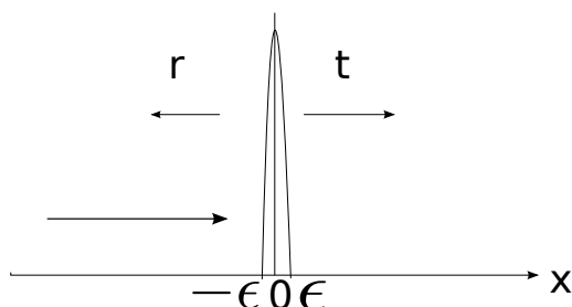
ABBILDUNG 1.10: Reflexion und Transmission am Deltapotential
