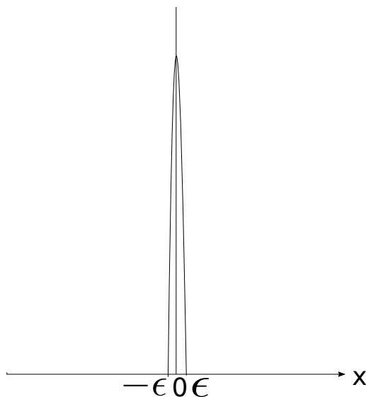
ABBILDUNG 1.9: Deltapotential
